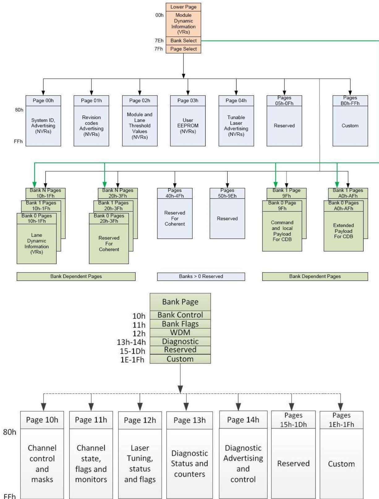
Figure4. QSFP DD Memory Map
