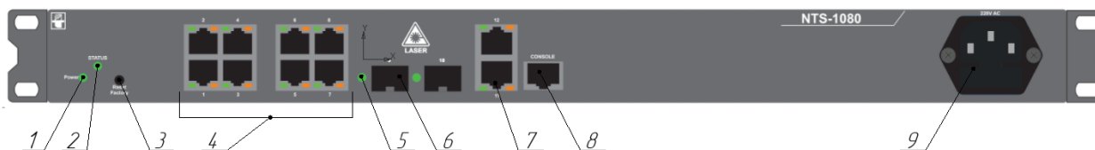
Рисунок 1.3.5 – Описание элементов лицевой панели NTS-1080
