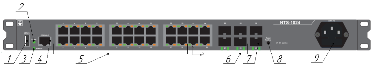
Рисунок 1.3.7 – Описание элементов лицевой панели NTS-1024/NTS-1024P
