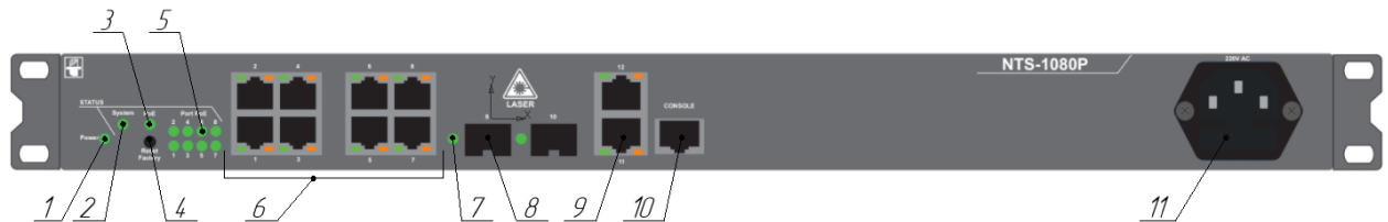
Рисунок 1.3.6 – Описание элементов лицевой панели NTS-1080P
