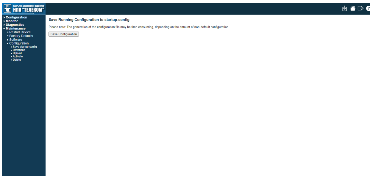
Рисунок 2.3.5 – Сохранение конфигурации
