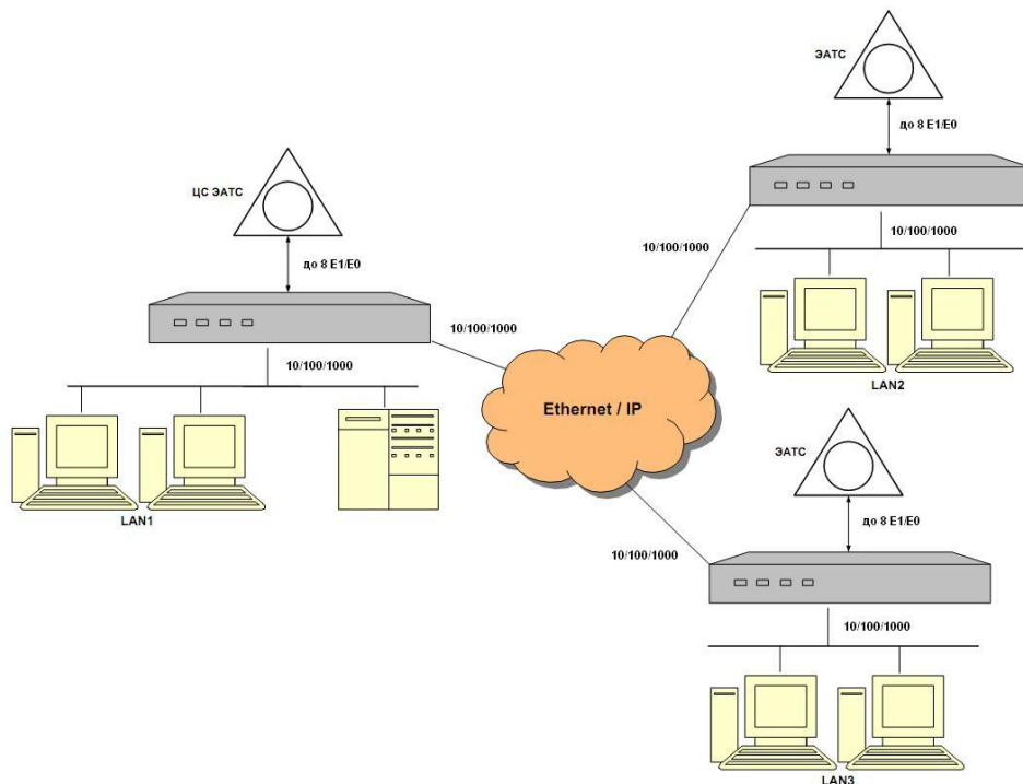
Схема 1 – Вариант построения сети на основе только мультиплексоров Оптик-4GE
