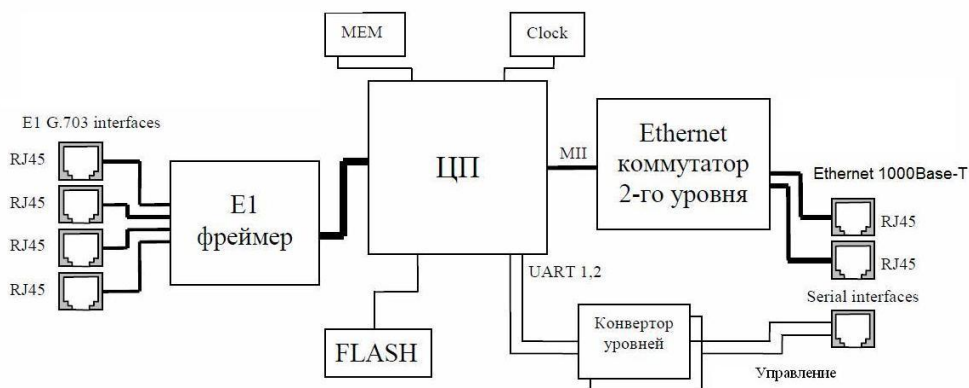
Рис. 2.5 - Внутреннее устройство блока
