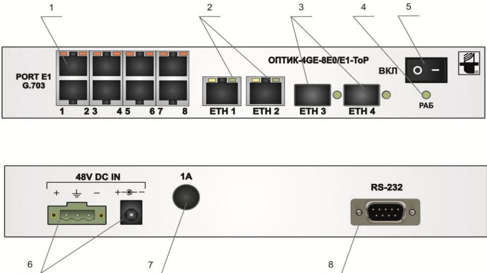
Рис. 1.13 - Внешний вид изделия Оптик-4GE-8E0/E1-ToP (mini)
