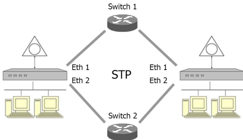
Схема 3 – Вариант построения кольцевой сети на основе протоколов STP
