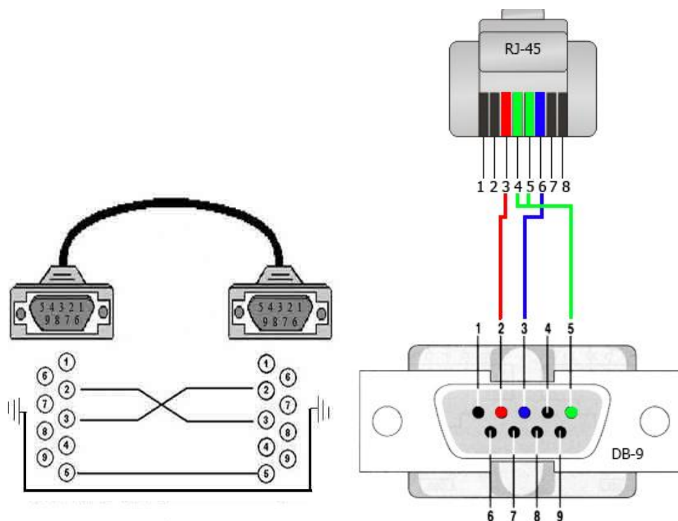
Рис. 3.3 - Схемы кабелей для подключения к блоку Оптик-4GE
