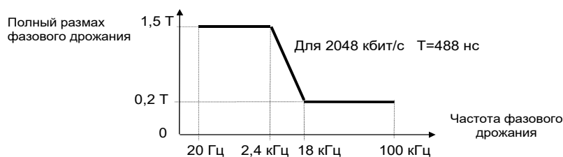
Рис. 2.1 - Нижний предел максимально допустимого фазового дрожания
