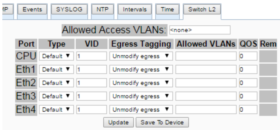
Рис. 3.42 – Вкладка Switch L2
