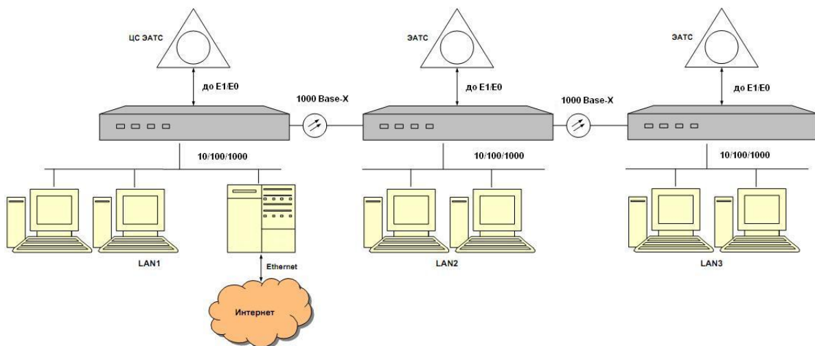
Схема 1 – Вариант построения сети на основе только мультиплексоров Оптик-4GE
